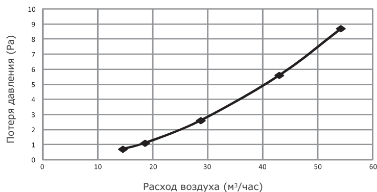
Потеря давления на 1 м длины трубки
